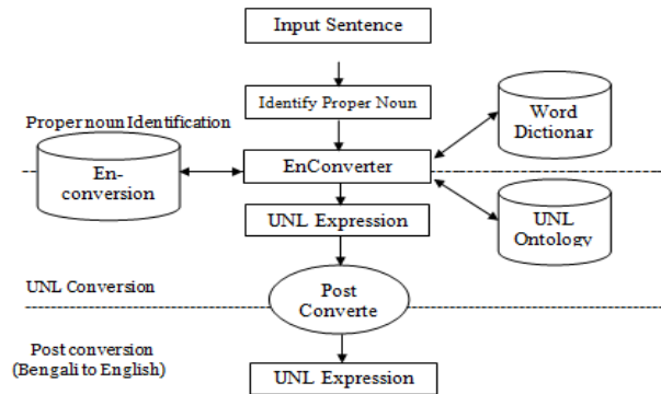
Figure 2. Flow chart of proper noun (নাম বাচক বিশেষ্য পদ) conversion
